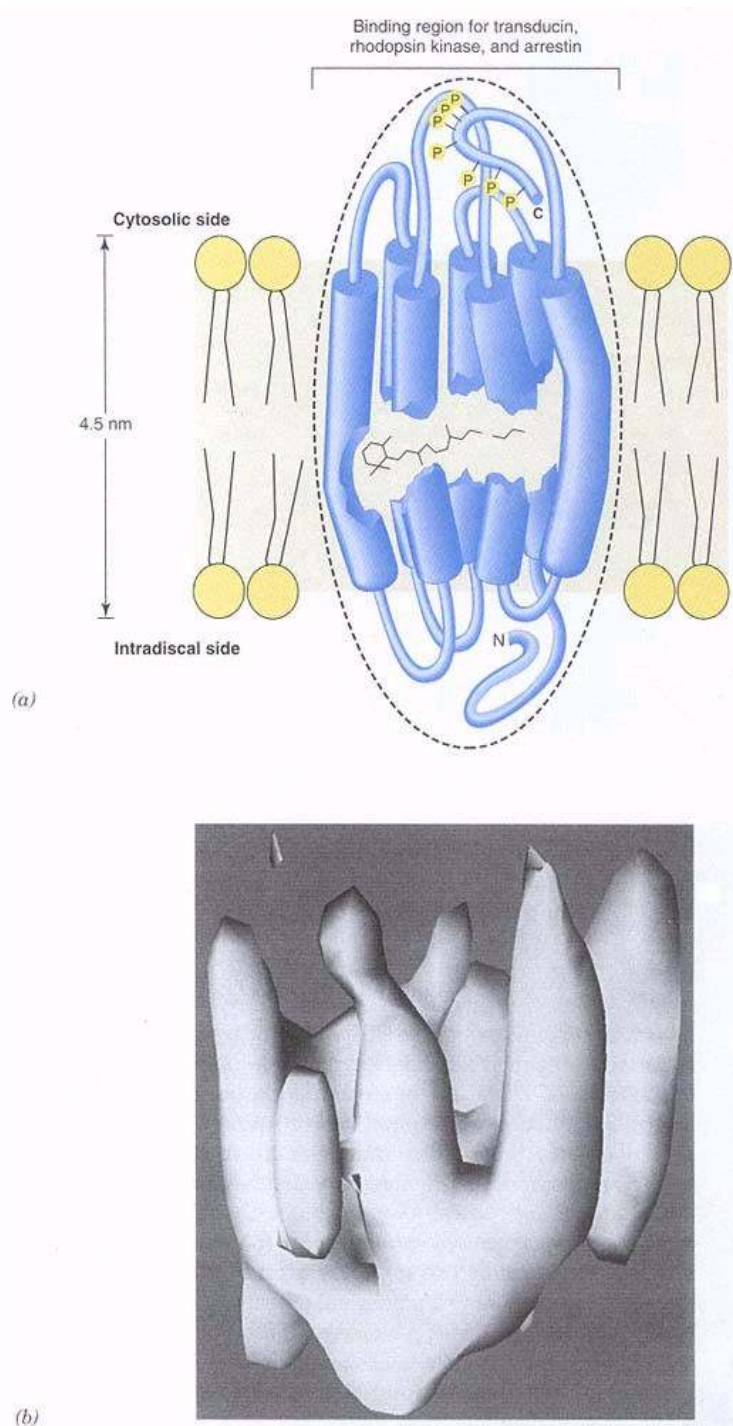
Figure 22.19 Rhodopsin.
